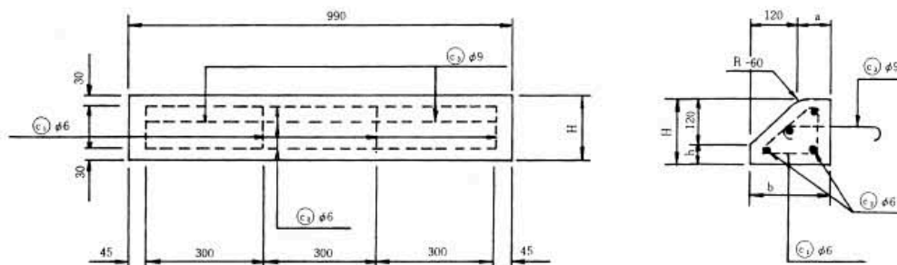
旧日本道路公団型 縁石PCC マウンタブル
