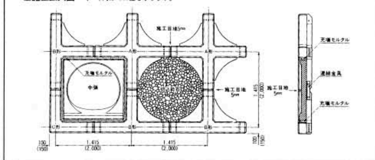
■施工拡大図 ( )内は500型を示します。
