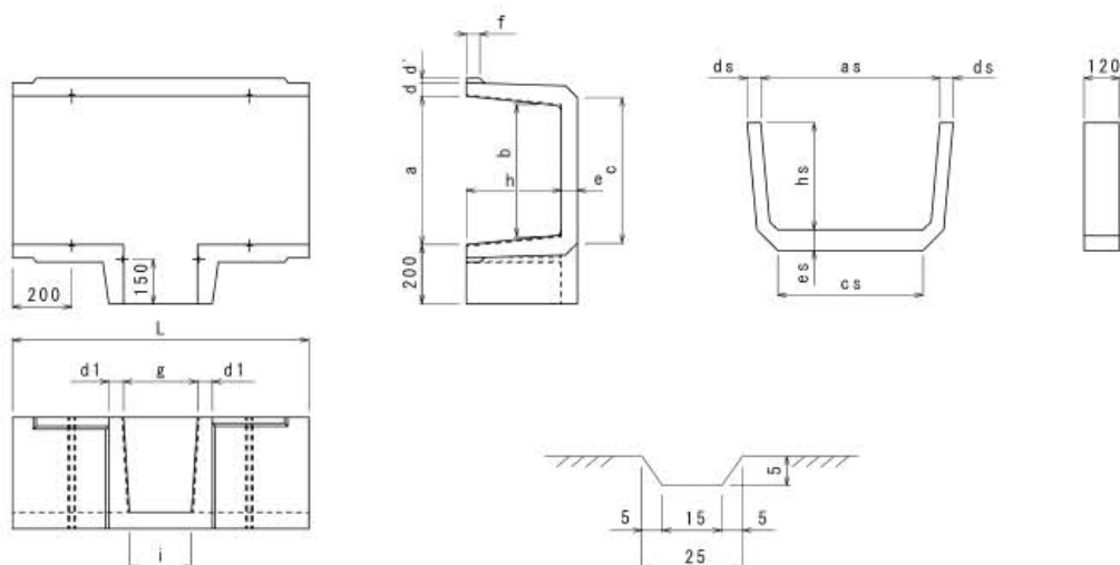
鉄筋コンクリートベンチフリューム用分水
