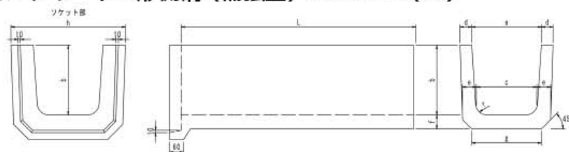
旧日本道路公団型 プレキャストコンクリートU形側溝
