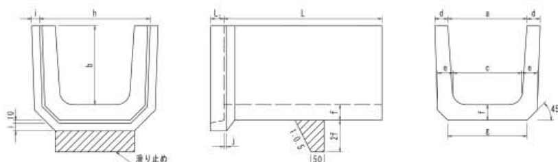
旧日本道路公団型 ソケット付U形側溝
