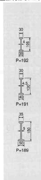
主部材形状・ピッチ
