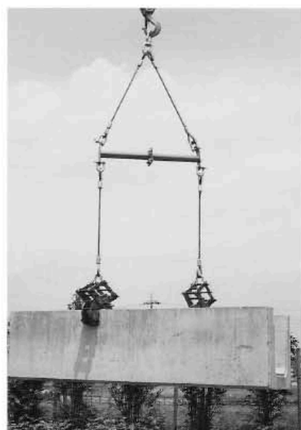
バランスアーム L-80
