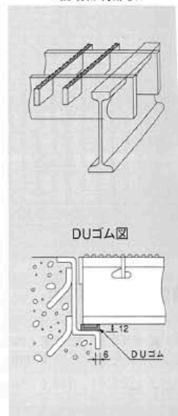
補助部材形状
