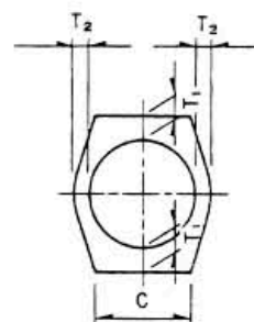
t-t断面図
