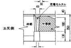
■連結詳細図
