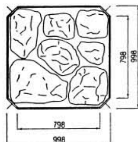
寸法表(mm)
