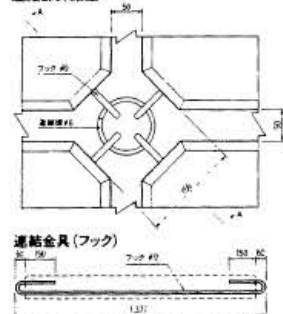
連結部詳細図
