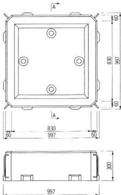
規格諸元
