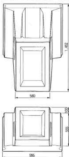
銀鱗Ⅳ型 1.5割 A形
