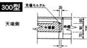
■充填部拡大図
