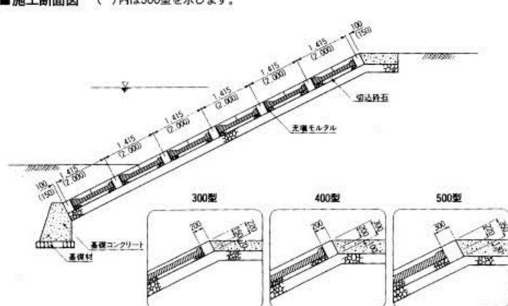
■施工断面図 ( )内は500型を示します。
