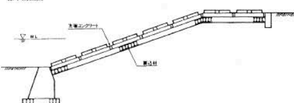
標準断面図
