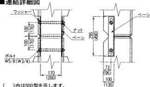
■連結詳細図
