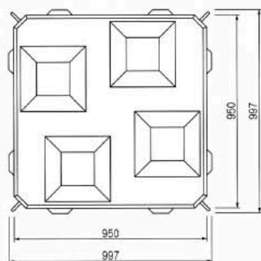
■規格寸法図
