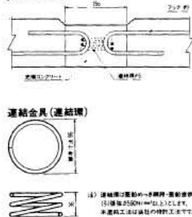
A-A断面図
