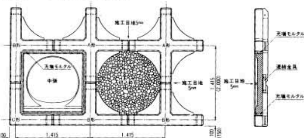
■施工拡大図 ( )内は 500型を示します。
