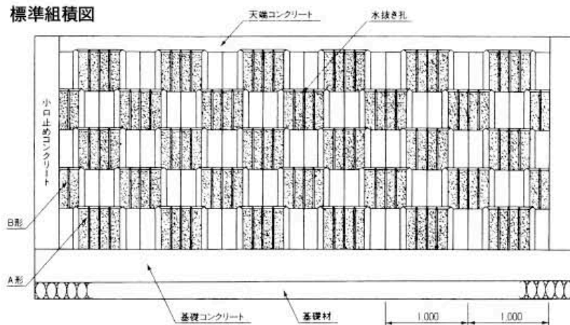
標準組積図
