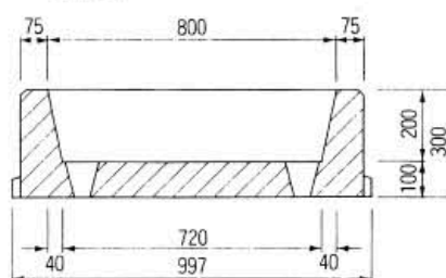
A-A断面図
