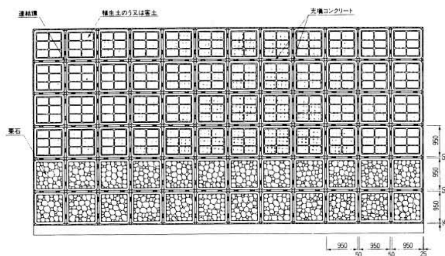
■標準断面図
