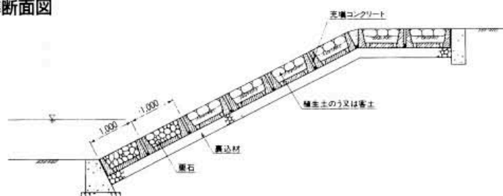
■標準断面図
