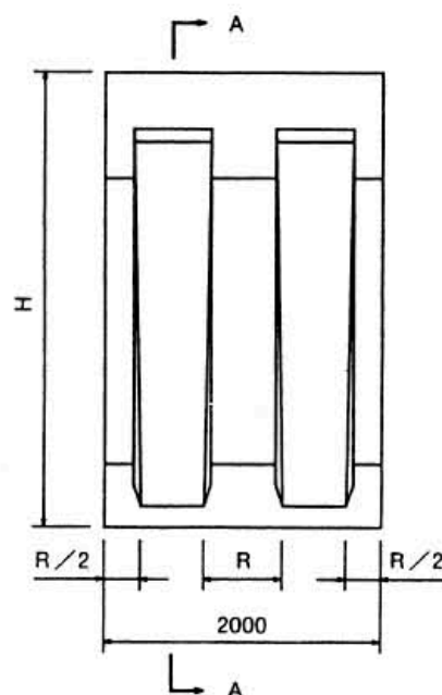
背面図
