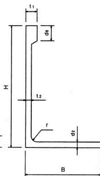
断面A-A
